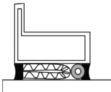
Figur 11. Oisolerad karm, E-klass
