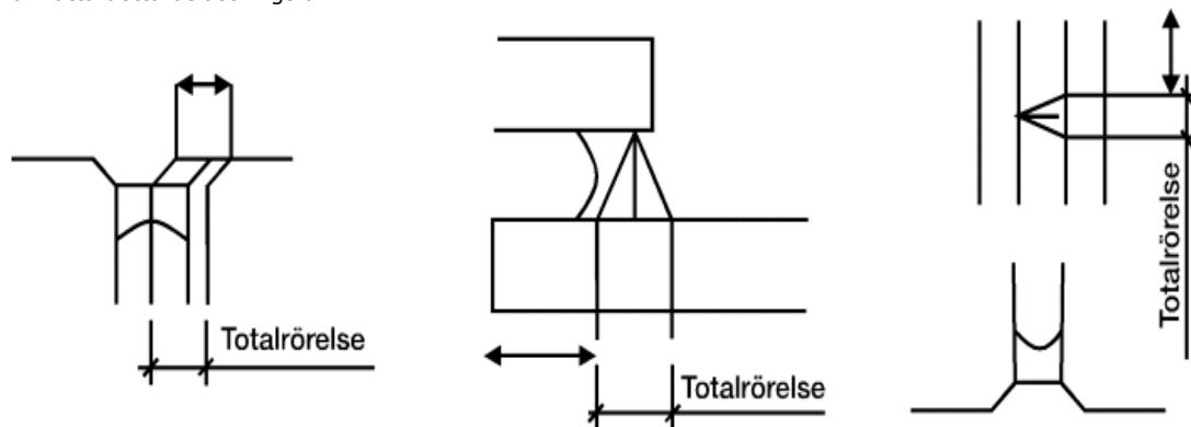
Figur RA Z/1, utdrag ur RA93 Hus
